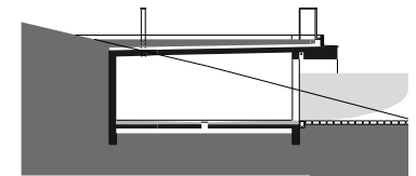
SCHNITT A-A
