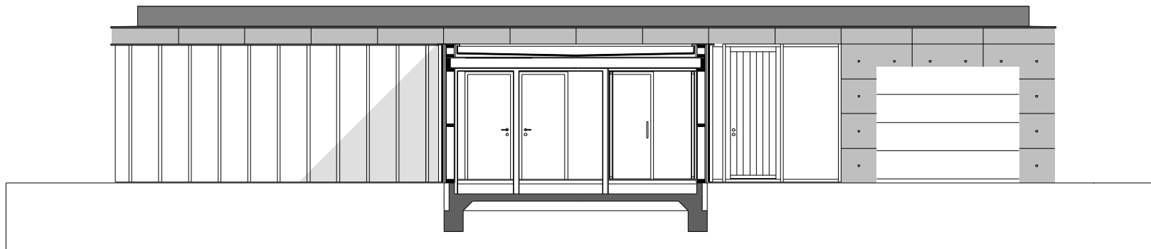
SCHNITT 2-2
