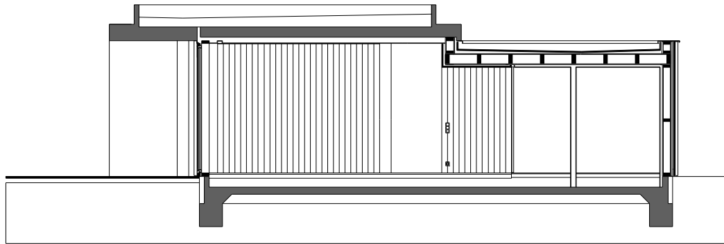
SCHNITT 1-1
